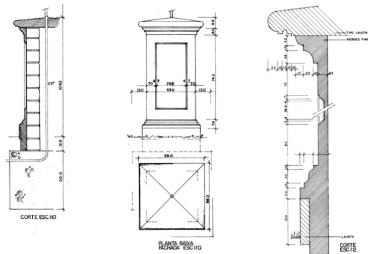
Detailzeichnungen
