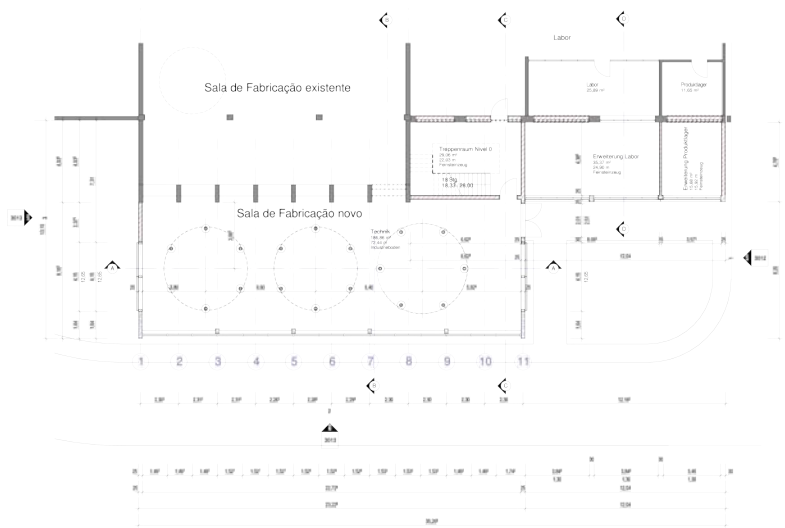
Planausschnitt
